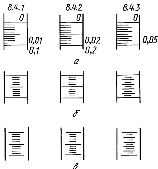
a — схема градуировки 1 (см. п. 8.3.1); б — схема градуировки 2 (см. п. 8.3.2); в — схема градуировки 3 (см. п. 8.3.3)
